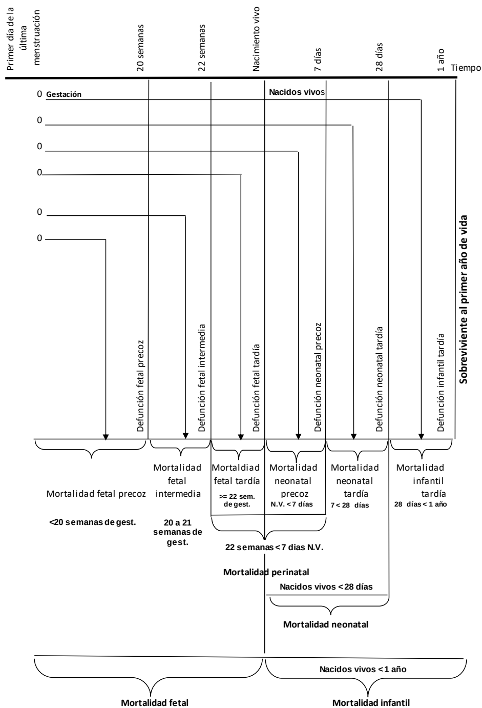
Diagrama 3: Cuadro esquemático de mortalidad fetal, neonatal e infantil
