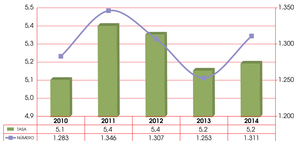
GRÁFICO 14: Defunciones neonatales, nivel país en número y tasa, período 2010-2014
